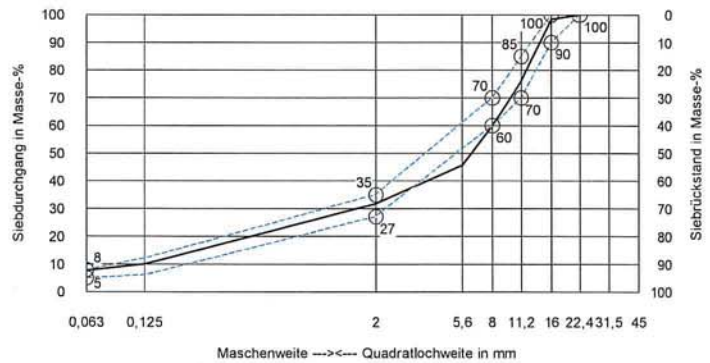
Sieblinienbereich für AC 16 B S SG
