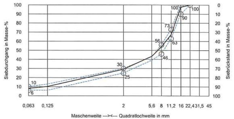
Sieblinienbereich für SMA 16 B S
