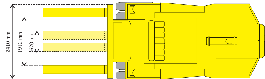
Variante 2: Gabeln
