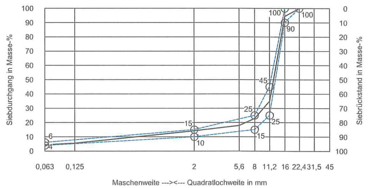
Sieblinienbereich für PA 16 T WDA MVV 2013
