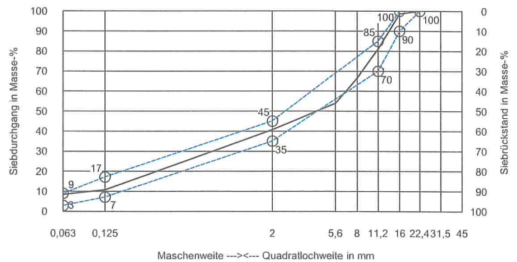
Sieblinienbereich für AC 16 D S
