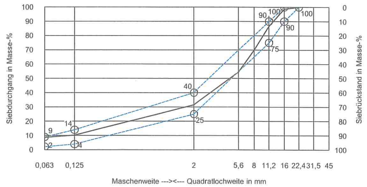
Sieblinienbereich für AC 16 T S
