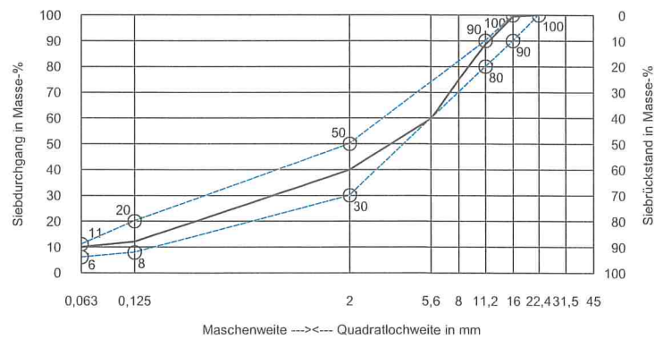
Sieblinienbereich für AC 16 TD LW
