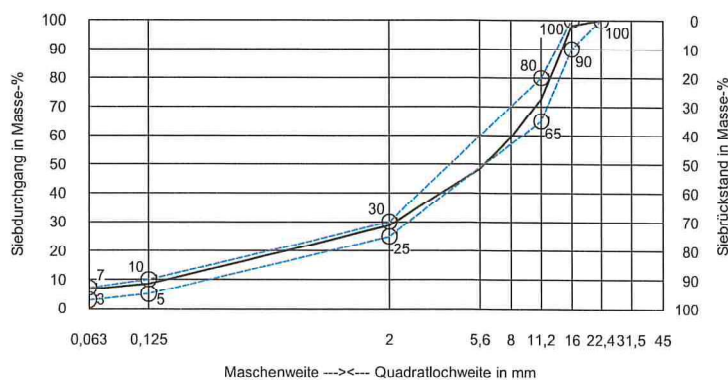
Sieblinienbereich für AC 16 B S
