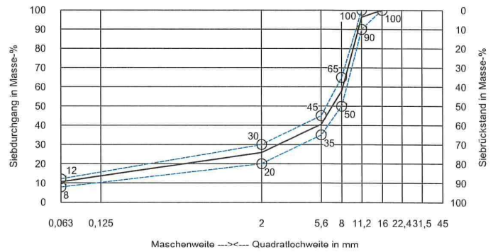
Sieblinienbereich für SMA 11 S
