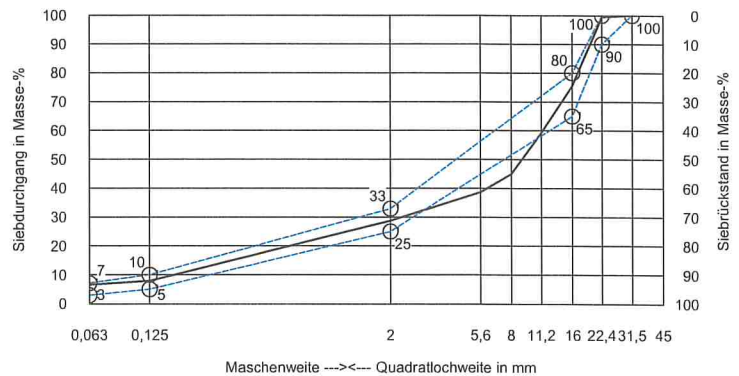
Sieblinienbereich für AC 22 B S
